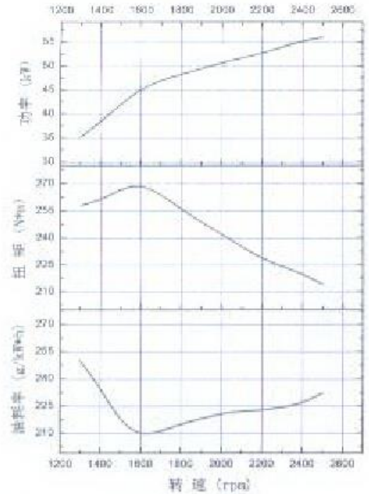
F4L914性能曲线
